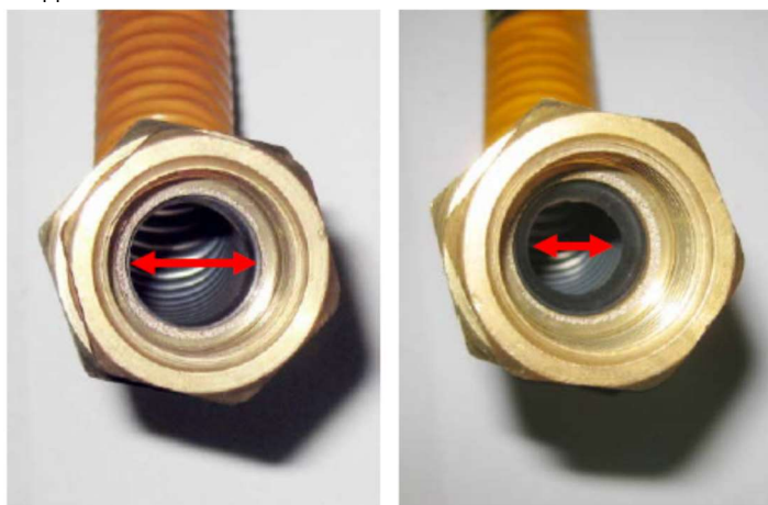
< Проверка уплотнения соединения впускной трубы газа >
